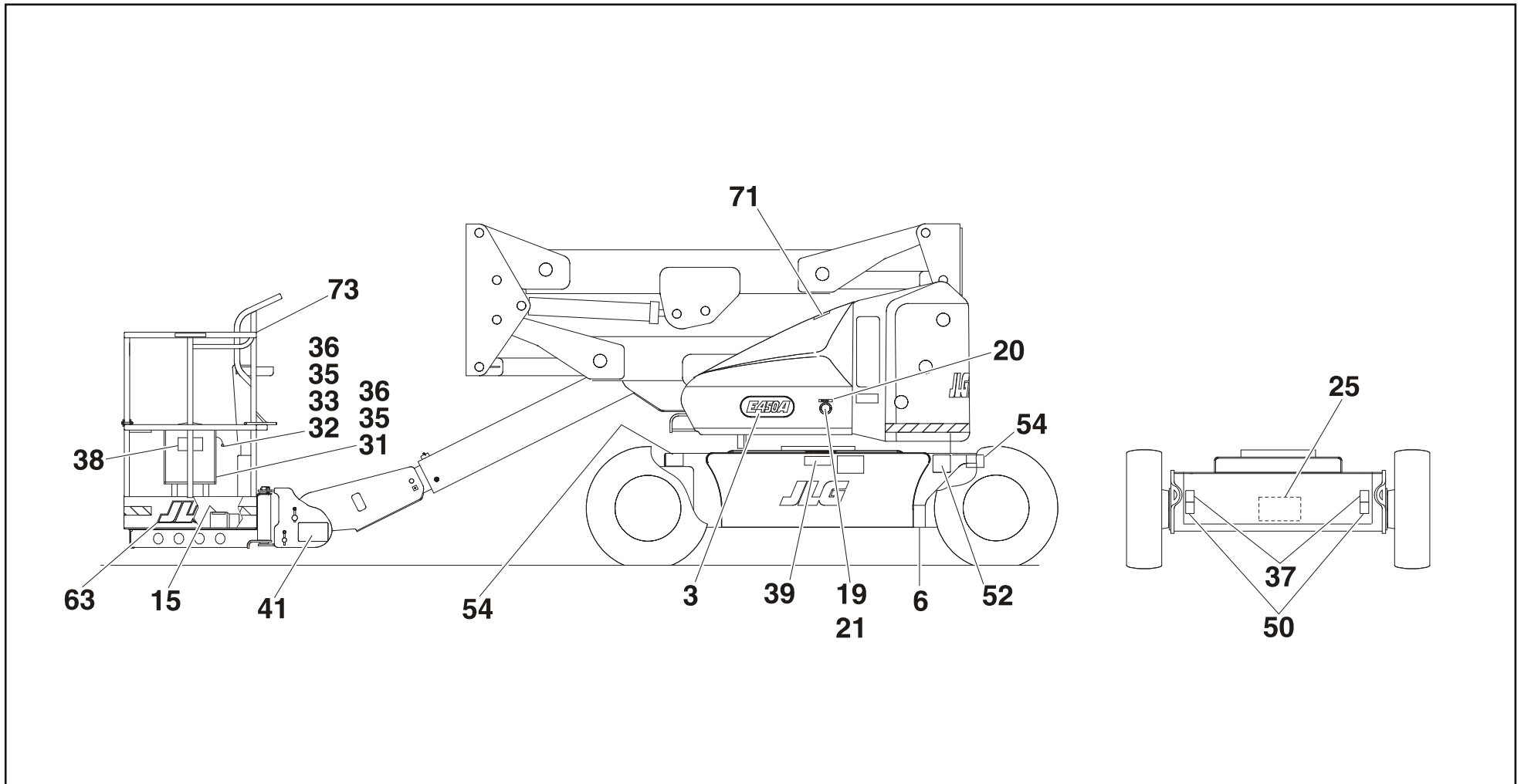
Figura 4-7. Instalación de etiquetas - Hoja 3 de 3
