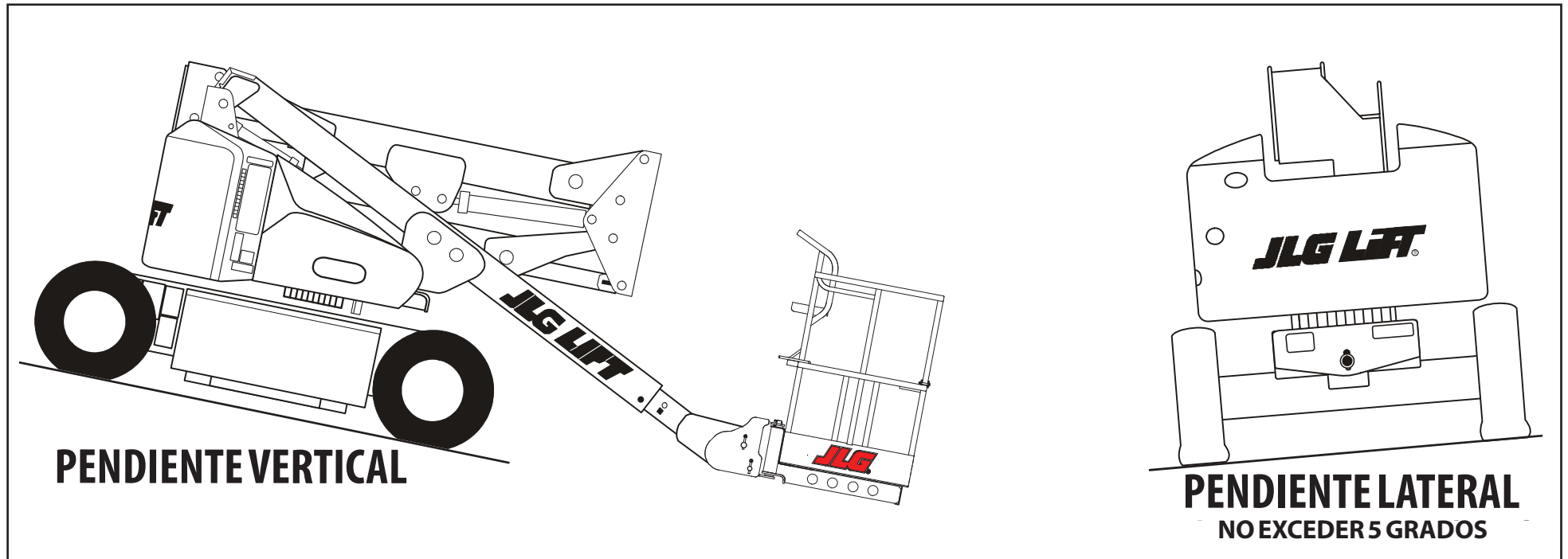
Figura 4-3. Pendientes verticales y laterales
