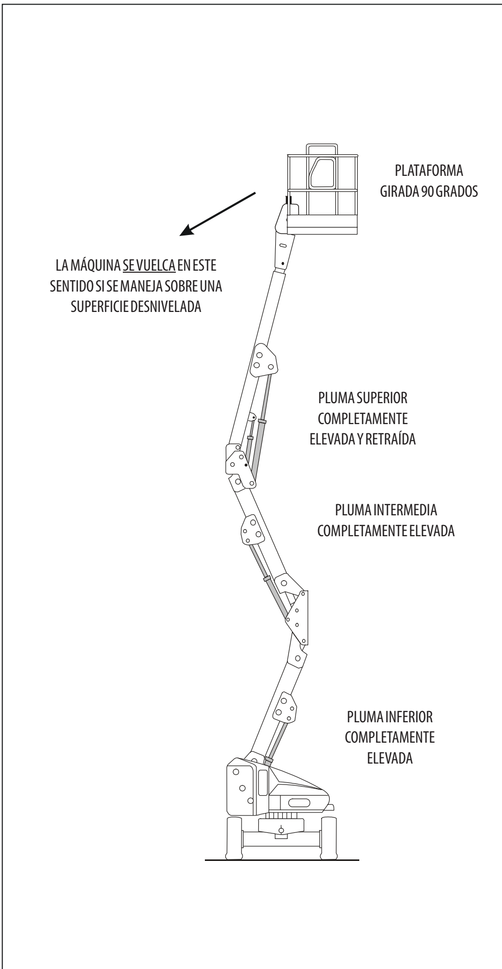
Figura 4-2. Posición de estabilidad trasera mínima
