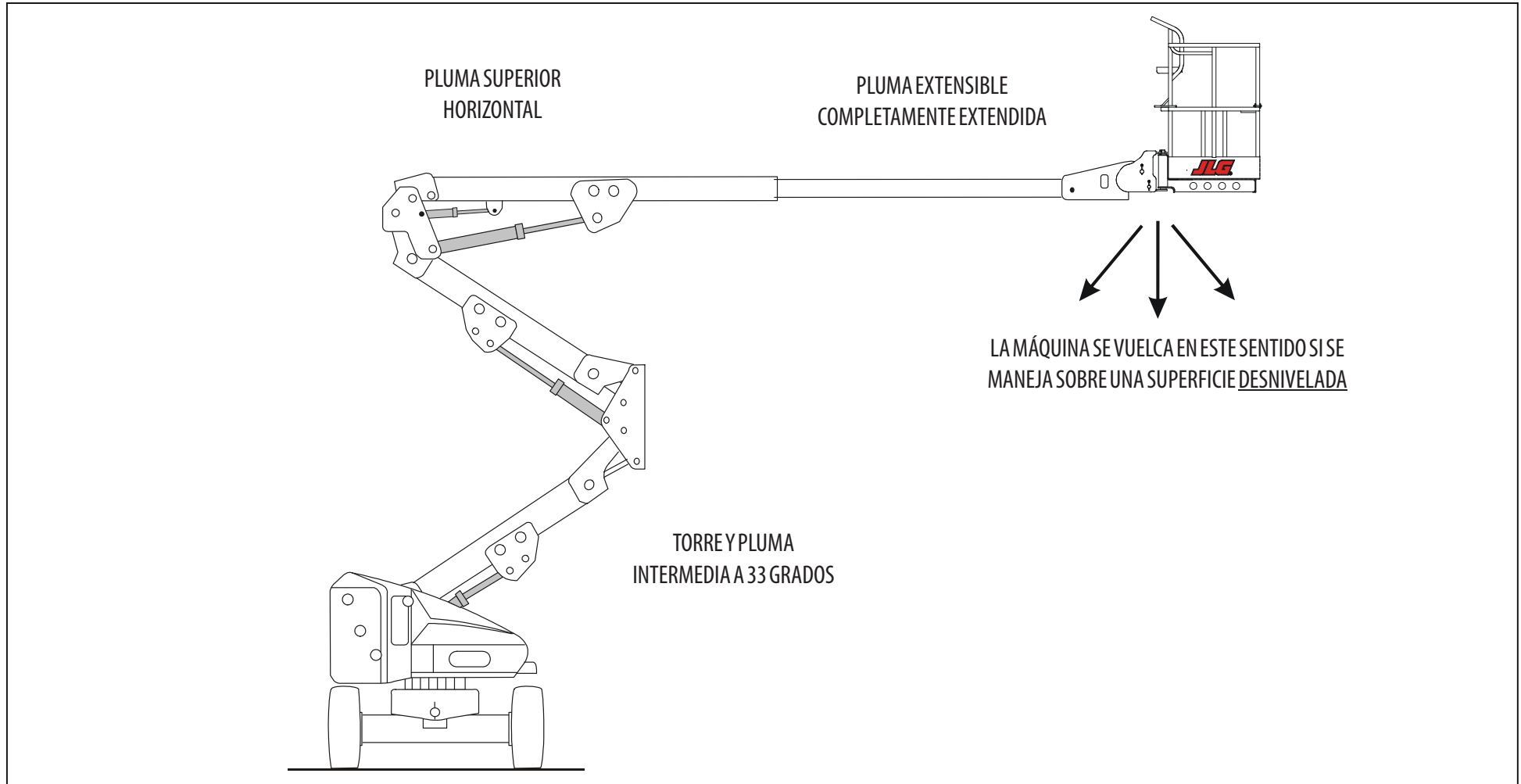
Figura 4-1. Posición de estabilidad delantera mínima
