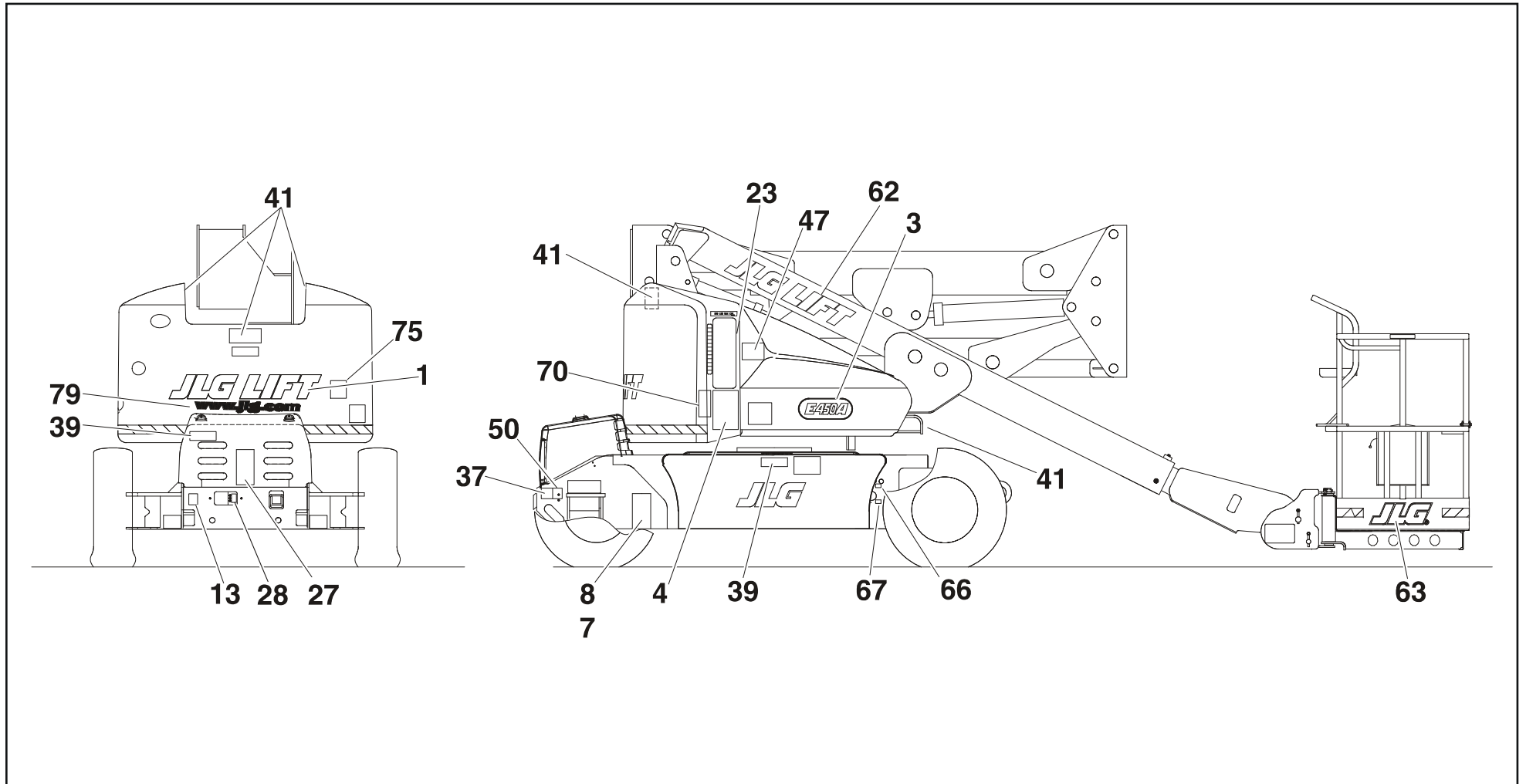
Figura 4-5. Instalación de etiquetas - Hoja 1 de 3
