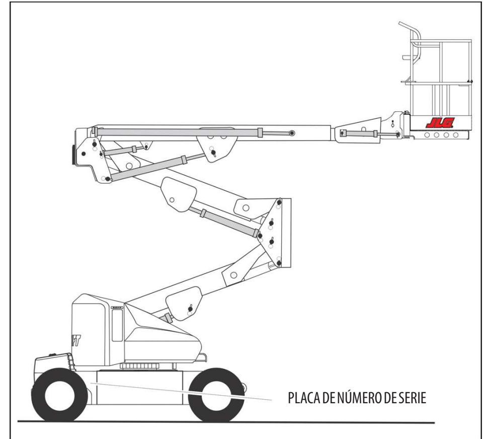
Figura 6-1. Ubicaciones del número de serie
