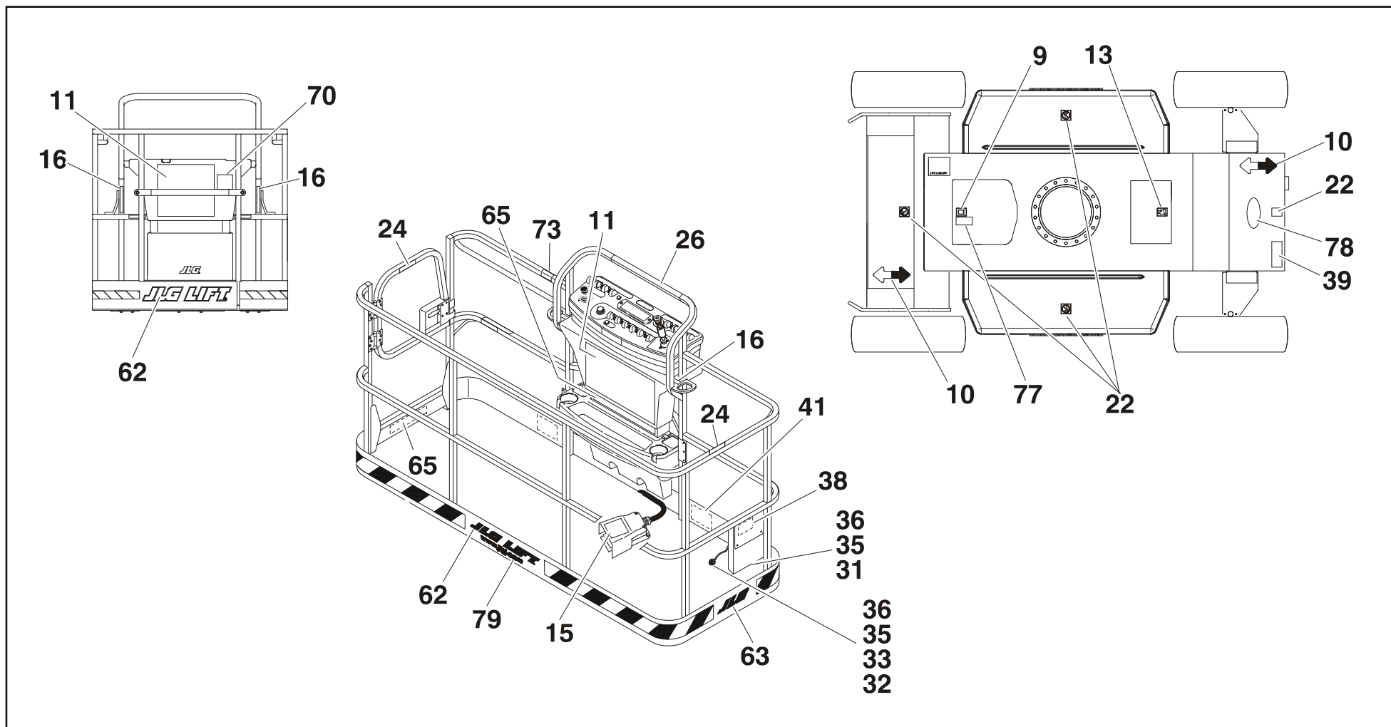
Figura 4-6. Instalación de etiquetas - Hoja 2 de 3
