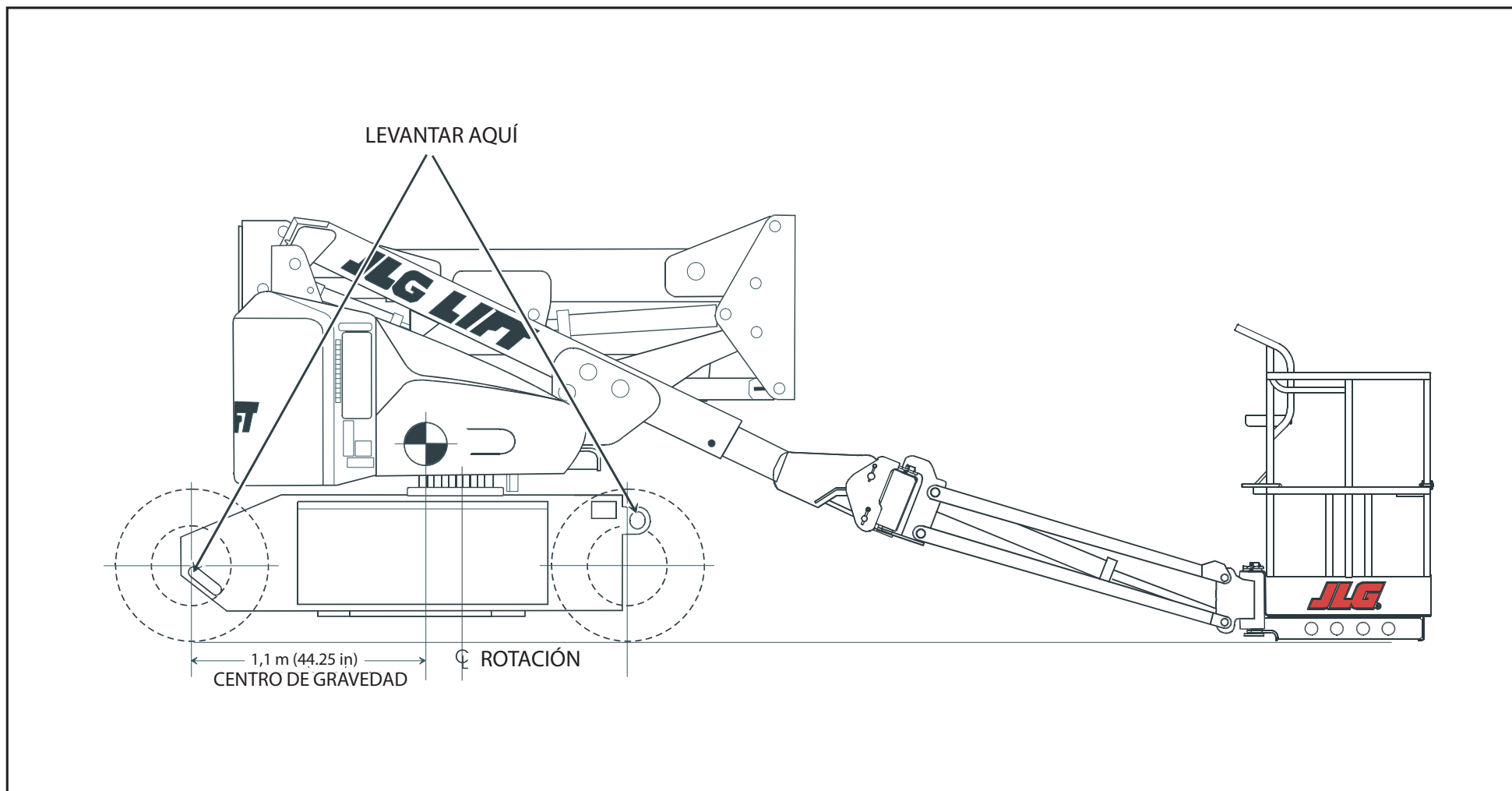
Figura 4-4. Tabla de levante
