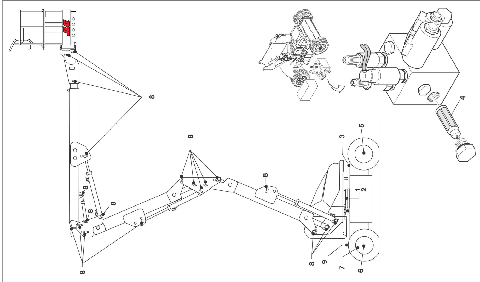
Figura 6-3. Diagrama de mantenimiento y lubricación de la M400
