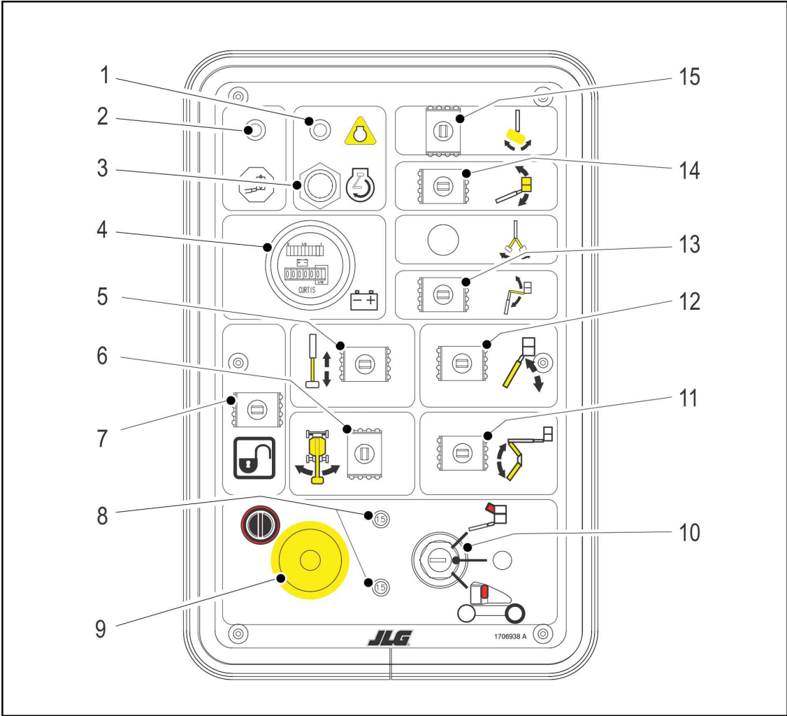
Figura 3-1. Puesto de controles de suelo
