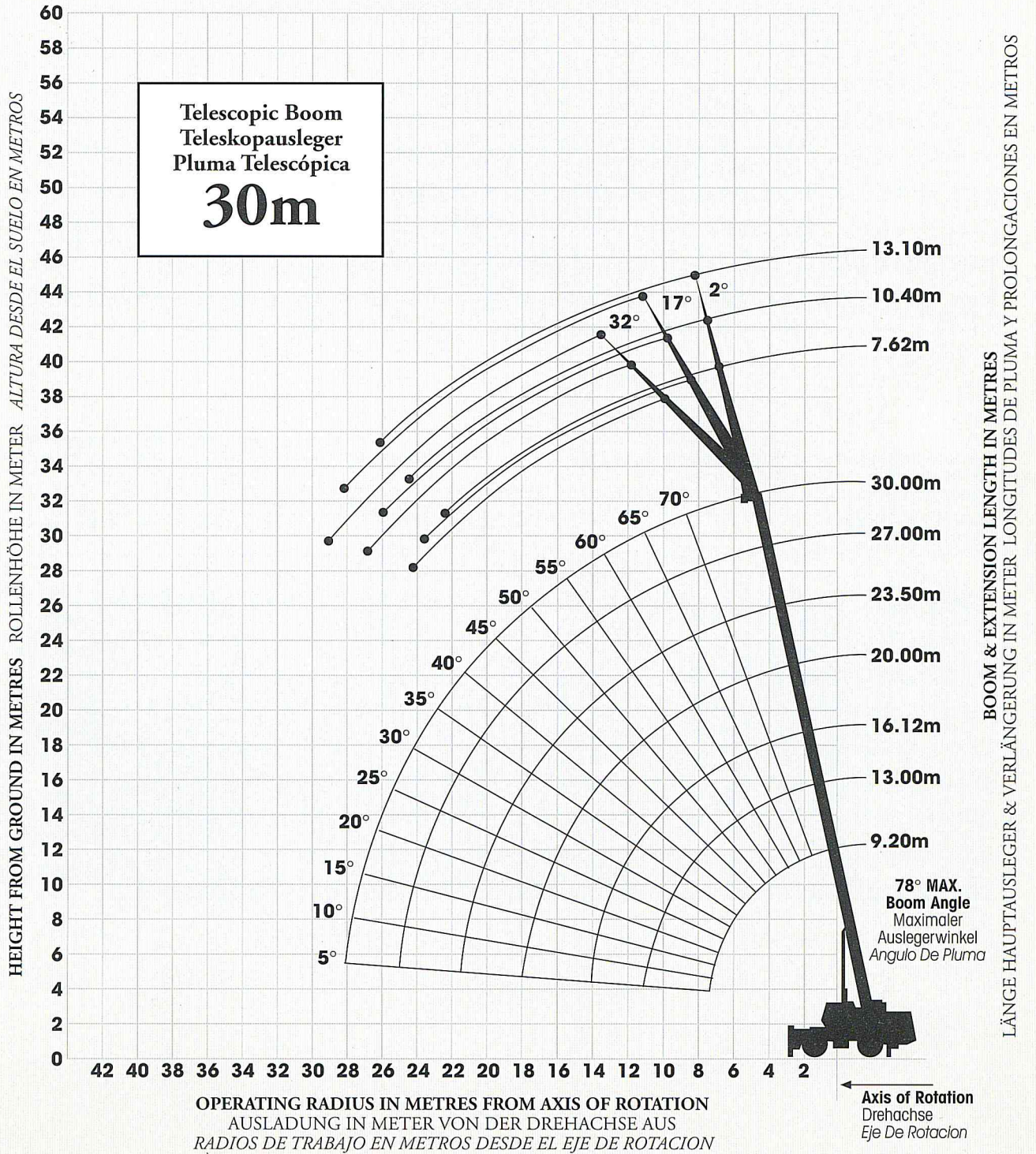
WORKING RANGE DIAGRAM ARBEITSBEREICHSDIAGRAMM DIAGRAMA DE ALCANCES
