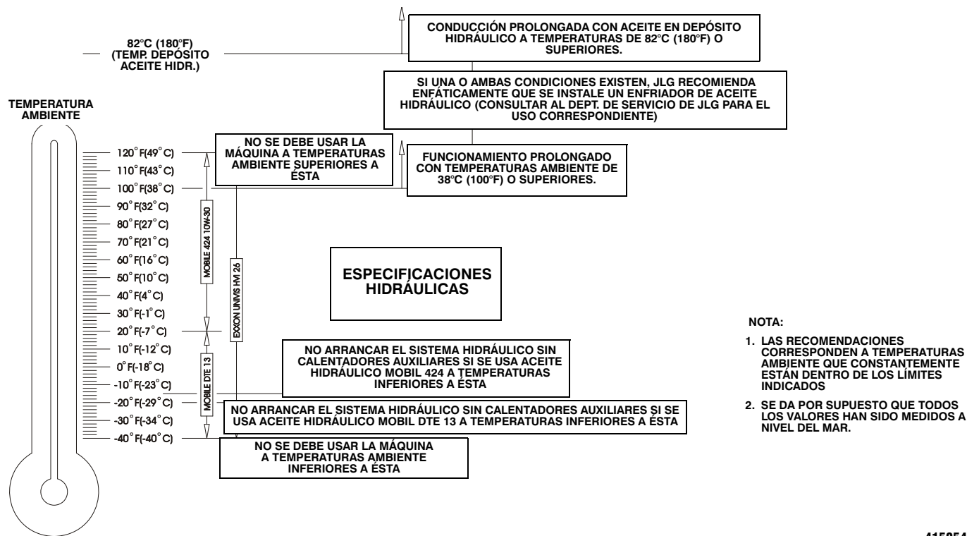
Figura 6-11. Especificaciones de temperaturas de funcionamiento del motor - Perkins - Hoja 2 de 2
