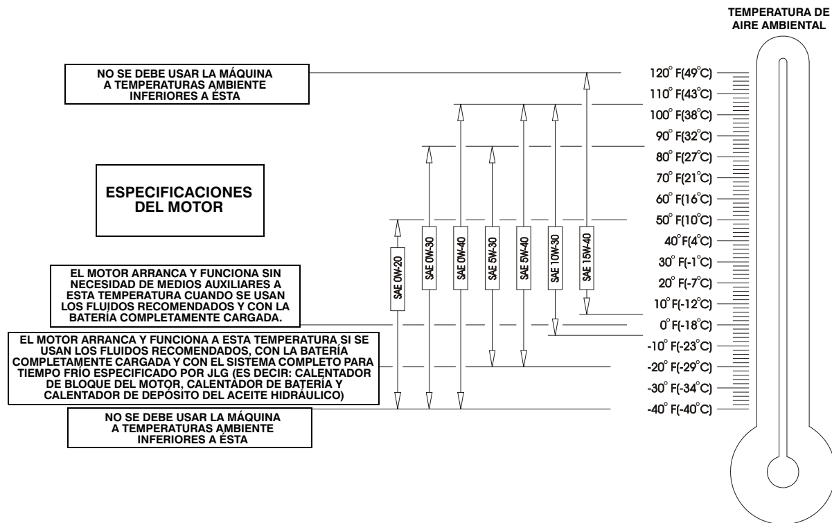
Figura 6-10. Especificaciones de temperaturas de funcionamiento del motor - Perkins - Hoja 1 de 2
