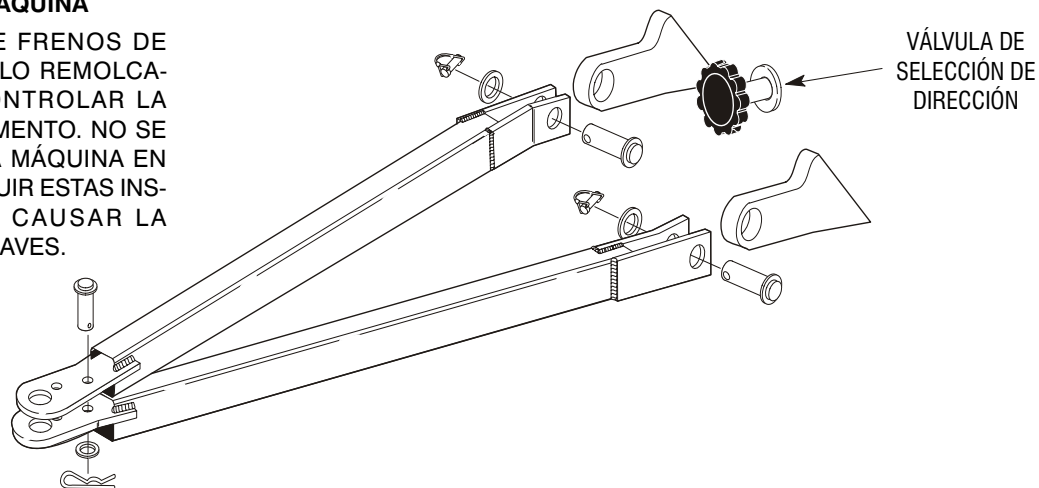
Figura 4-6. Puntos de conexión de barra de remolcado - Máquinas con NS 81836 al presente
