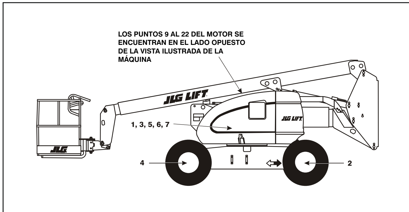
Figura 6-8. Puntos de lubricación y mantenimiento
