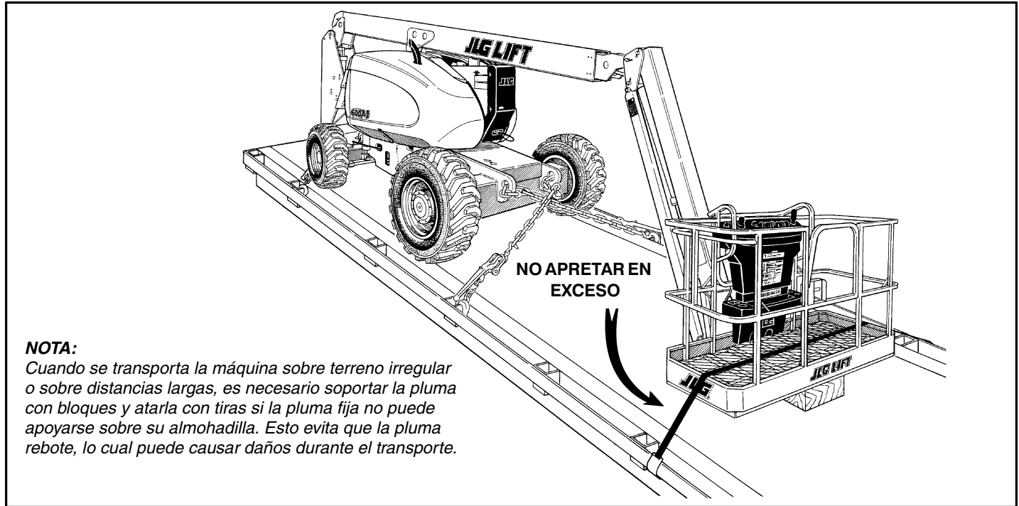
Figura 4-8. Amarre de la máquina
